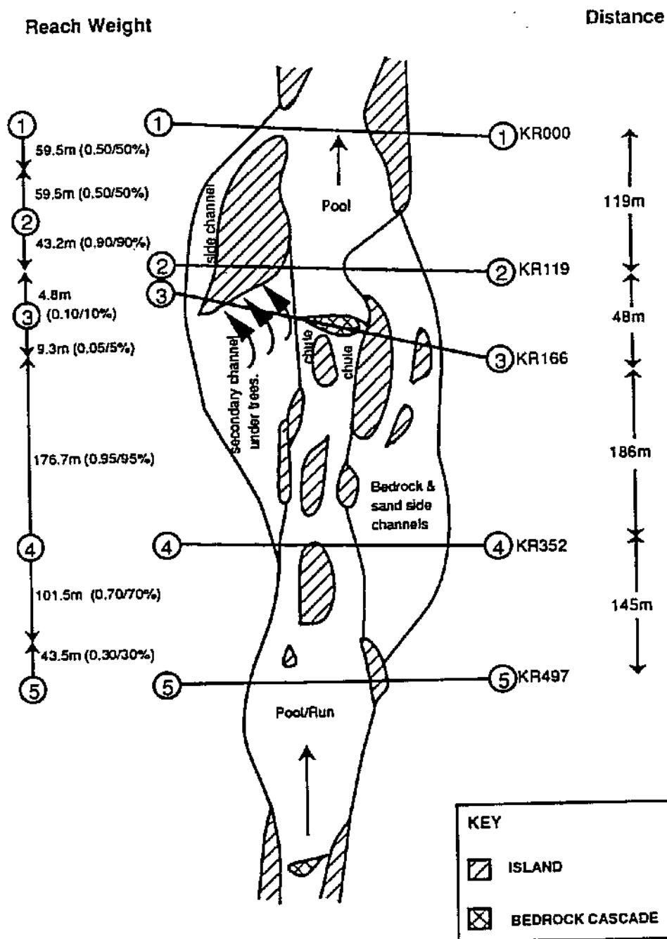
Figure 6.2 Site map of the PHABSIM II study site at Kriedouwkrans
