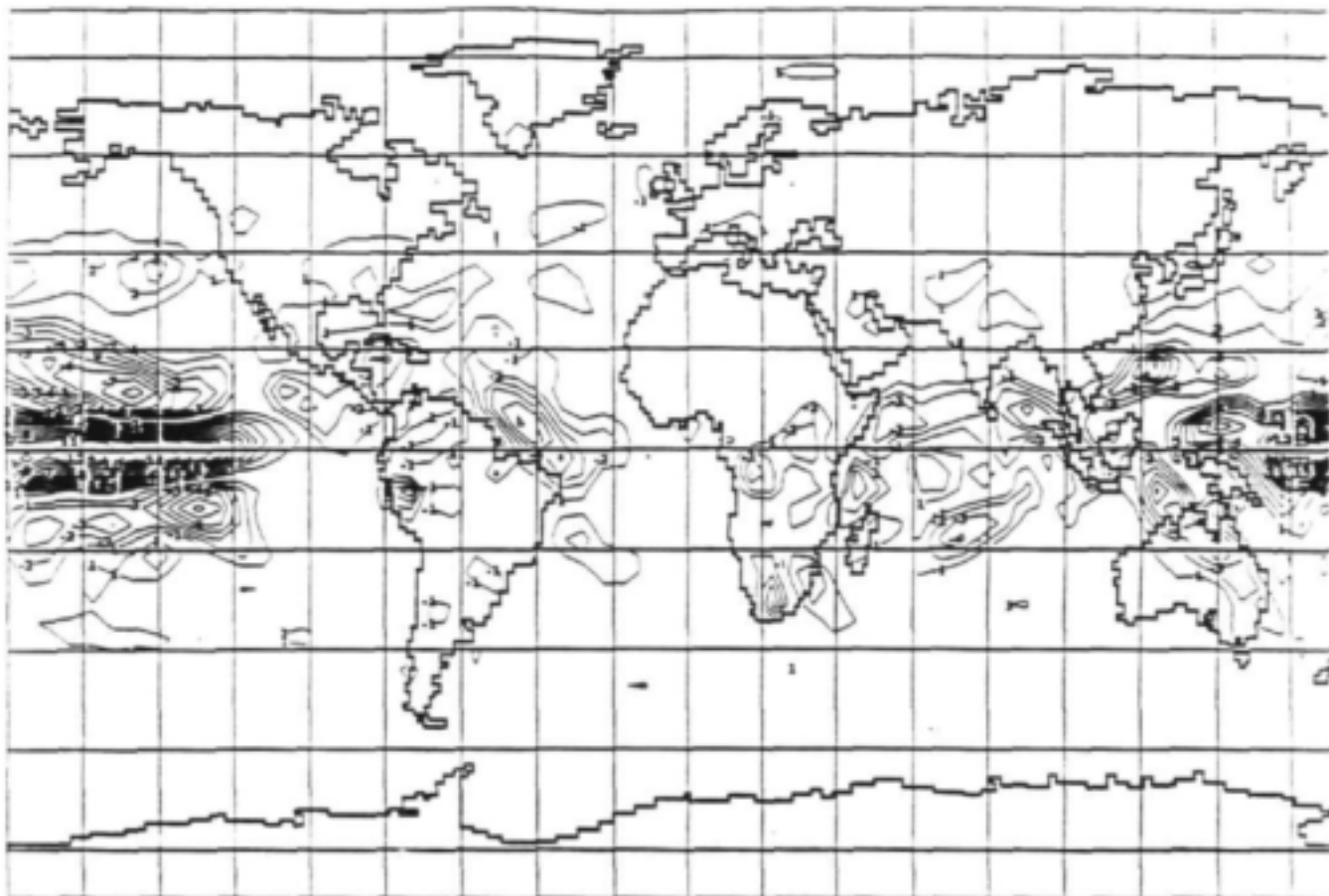
Figuur 17. CSIRO-4 model berekende reynval anomalie vir Desember in mm/dag. Die anomalie = +5^{\circ}\text{K} SOT anomalie lopie minus die kontrole lopie (Eksperiment 2).
