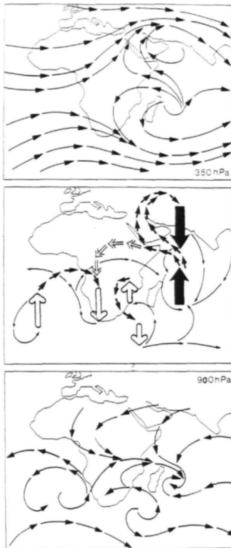
Figuur 25. 'n Onedimensionele voorstelling van die sirkulasie patrone vir die 6°K SOT anomale "dipool" eksperiment (Eksperiment 2). Die boonste skets dui op die primêre 350 hPa drukvlak horisontale windveld. Die onderste skets is dieselfde maar vir die 900 hPa drukvlak. Die middelste skets is 'n voorstelling van die vertikale beweging (dik swart pyl) sowel as die sekondêre sirkulasie op die 350 hPa drukvlak (dun swart lyn) en die sekondêre sirkulasie (dun stippel lyn) op die 900 hPa drukvlak. Die oop pyl dui sekondêre sirkulasie vanaf die suid-wes Indiese oseaan via ekwatoriaal Afrika na Suid Afrika aan.
