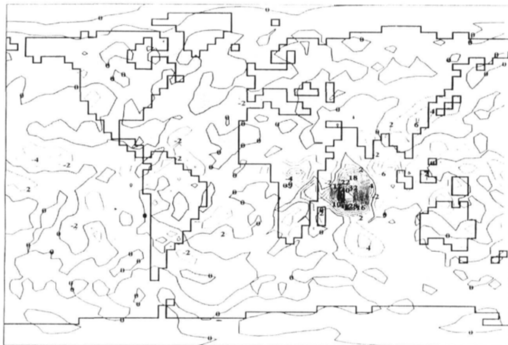
Figuur 13. CSIRO-4 model berekende reënval anomalië in mm/dag. Die anomalie = +5^{\circ}\text{K} SOT lopie reënval minus die reënval van die kontrole lopie (Eksperiment 1).
