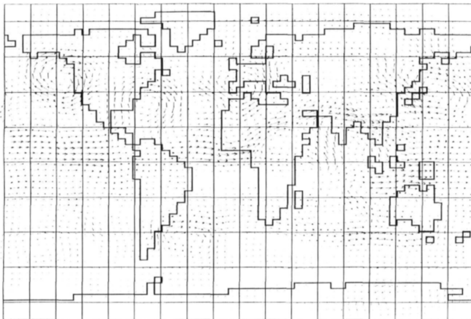
Figuur 11(c). Berekende 350 hPa drukvlak wind anomalie vir Februarie. Elke anomalie is die vektorverskil tussen die velde van fig.11(b) en fig.11(a) oftewel " +5^{\circ}\text{K} SOT lopie minus die kontrole lopie" (Eksperiment 1).
