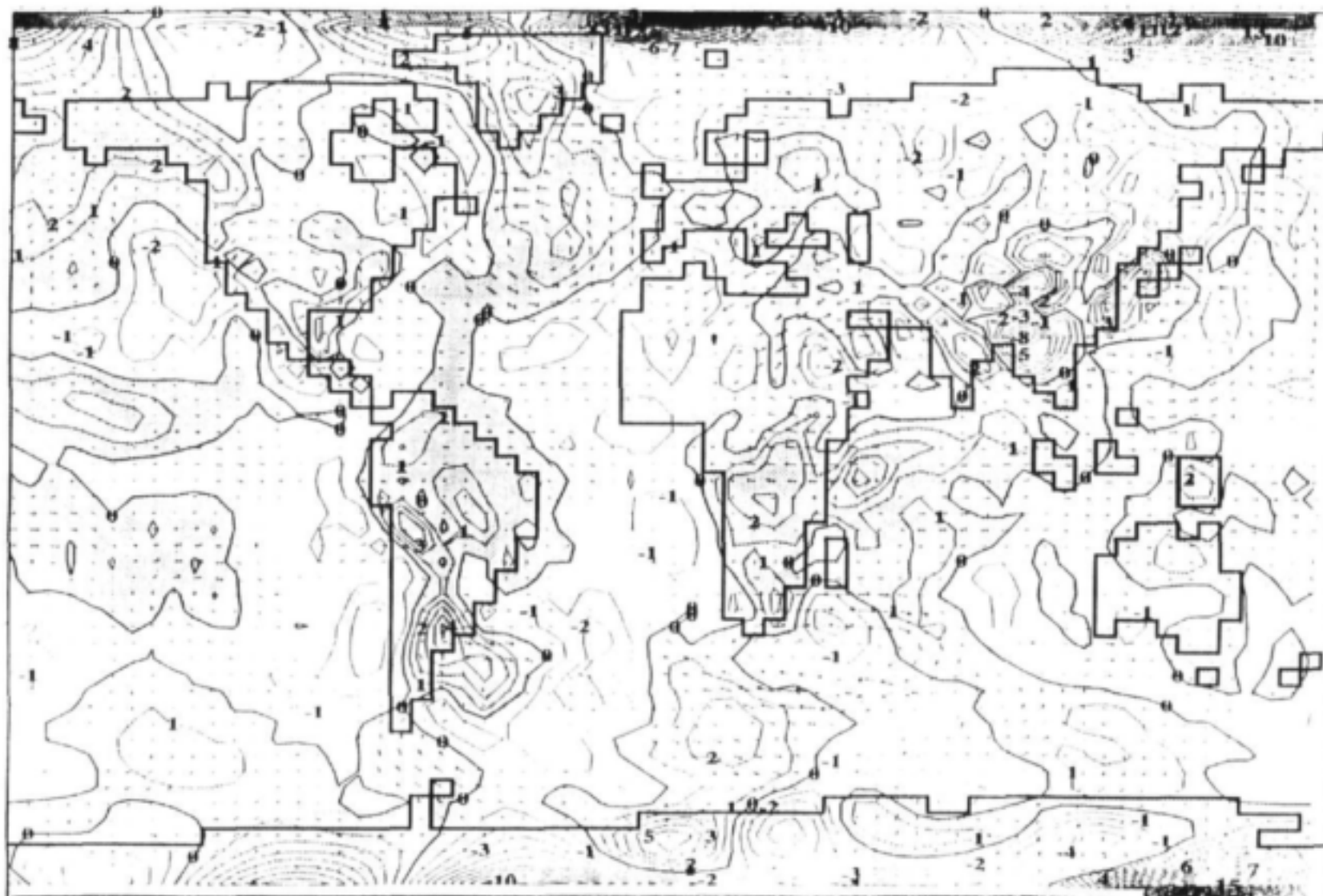
Figuur 22(a). CSIRO-4 model windvektor anomalie op die 350 hPa drukvlak vir Februarie uit die 'dipool' eksperiment met 'n 2^{\circ}\text{K} SOT anomalie (soos fig.21(a)). Die horisontale snelheidsdivergensie uitgedruk in (1 \times 10^6 \text{ m/s}) , en bereken uit die 350 hPa drukvlak windvektore van die 'dipool' eksperiment word op dieselfde drukvlak in kontoure
