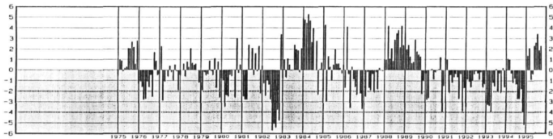
Figuur 2(a). 850 hPa drukvlak wind anomalië van die maandgemiddeld in m/s oor die westelike tropiese SO gedurende die periode 1975 tot 1995 (Positiewe anomalië verwys na 'n sterker as normale oostewind.)
