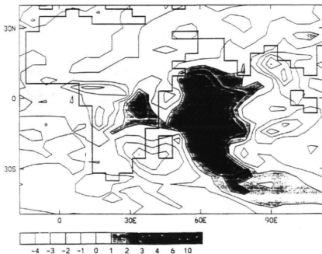
Figuur 27. CSIRO-9 model reënval anomalie data in (mm/dag) vir Februarie met 'n 2°K SOT anomalie noord-oos van Madagaskar (Eksperiment 4).
