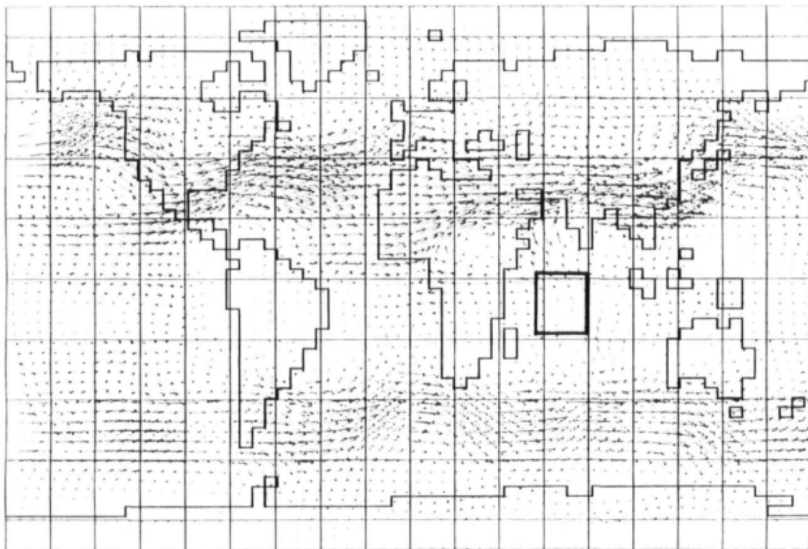
Figuur 11(b). Soos fig.11(a) maar uit die CSIRO-4 model met 'n +5^{\circ}\text{K} SOT anomalie noord-oos van Madagaskar. Die areas met 'n +2^{\circ}\text{K} en +5^{\circ}\text{K} anomalie is ingeteken met dik swart lyne (Eksperiment 1).
