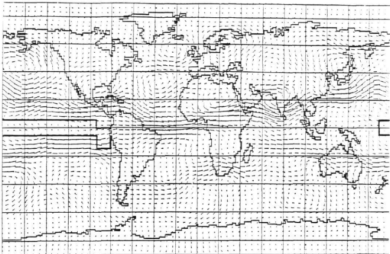
Figuur 15. CSIRO model berekende wind vektor anomalië in m/s op die 350 hPa drukvlak vir Desember. SOT anomalië van +5^{\circ}\text{K} oor die ekwatoriale SO word met dik swart lyne aangedui (Eksperiment 2).
