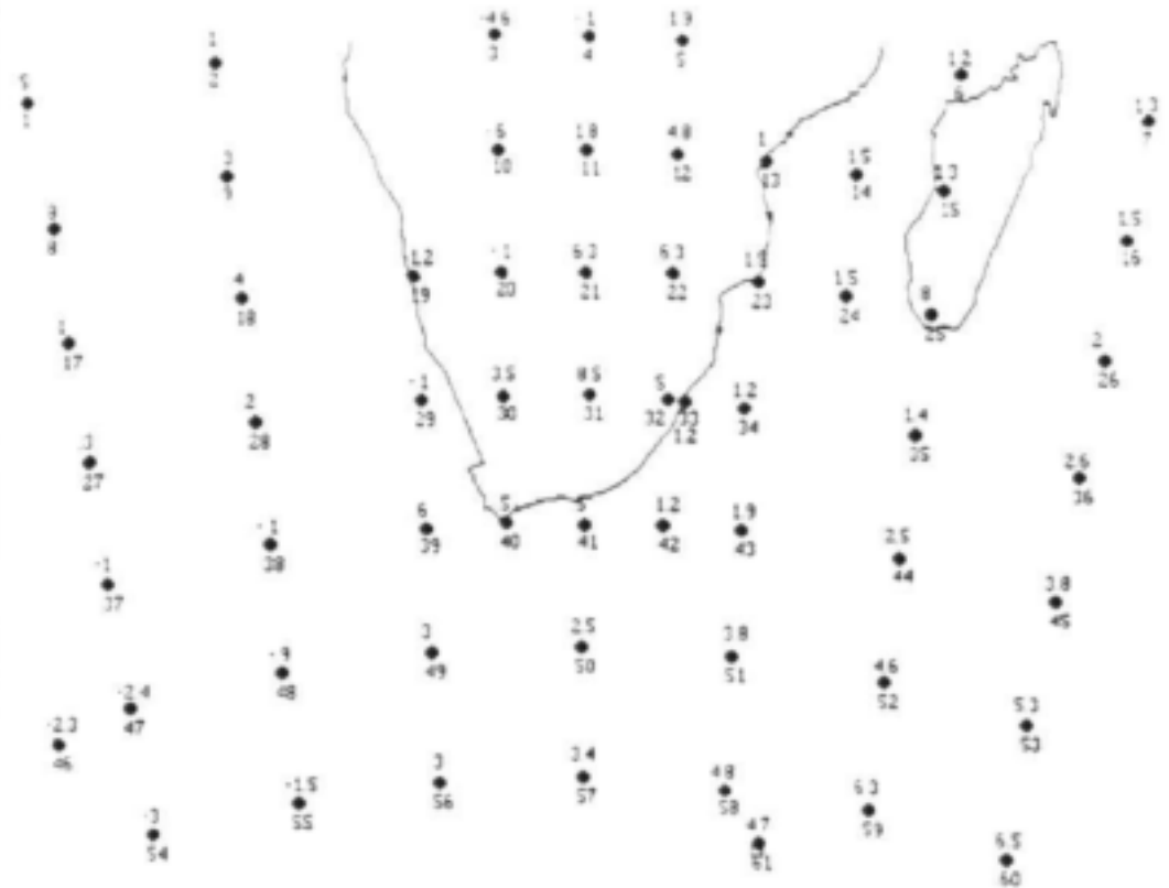
Figuur 28. Die geografiese ligging van die roosterpunte benut vir die versyfering van die daaglikse weerbulletin.
