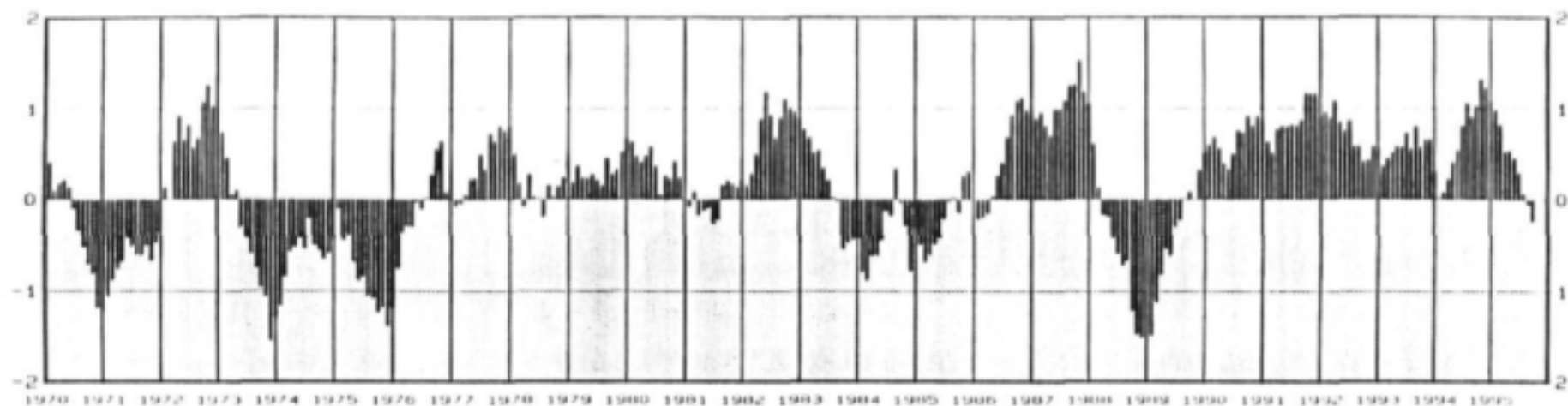
Figuur 1(a). Maandgemiddelde See Oppervlak Temperatuur (SOT) anomalie in ( ^{\circ}\text{K} ) oor die tropiese Stille Oseaan (SO), of die Nino 4 gebied, gedurende die periode 1970 tot 1995.
