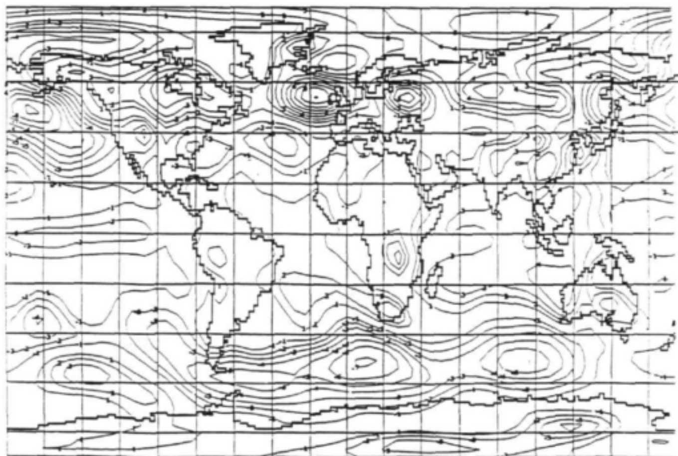
Figuur 18. CSIRO-4 model berekende oppervlak lugdruk anomalie in hPa vir Desember. Die anomalie = +5 SOT anomalie lopie minus die kontrole lopie (Eksperiment 2).
